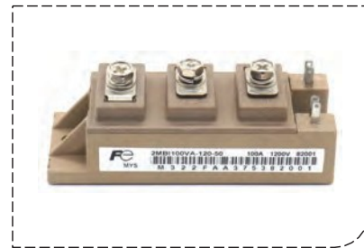
2MBI100VA-120-50 FUJI IGBT модуль
