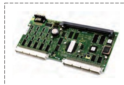
ID. NR. 591640 Schindler 5400 основная плата
