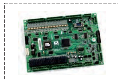
SM-01-F Step основная плата
