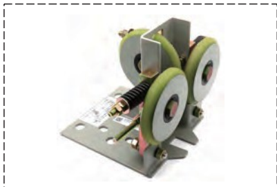
C0083111-B/16501278-A Hitachi башмак на роликах
