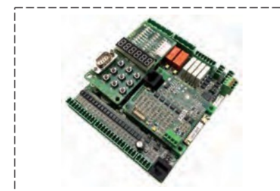
AS.T029 Step основная плата
