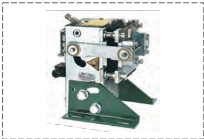
OX-250 ограничитель скорости
